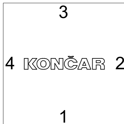
A Pogled X - Priklučni ormarić, položaj uvednica View X - Terminal box, cable gland position
