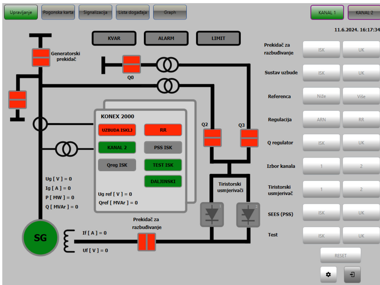
Korisničko sučelje za upravljanje sustava uzbude
