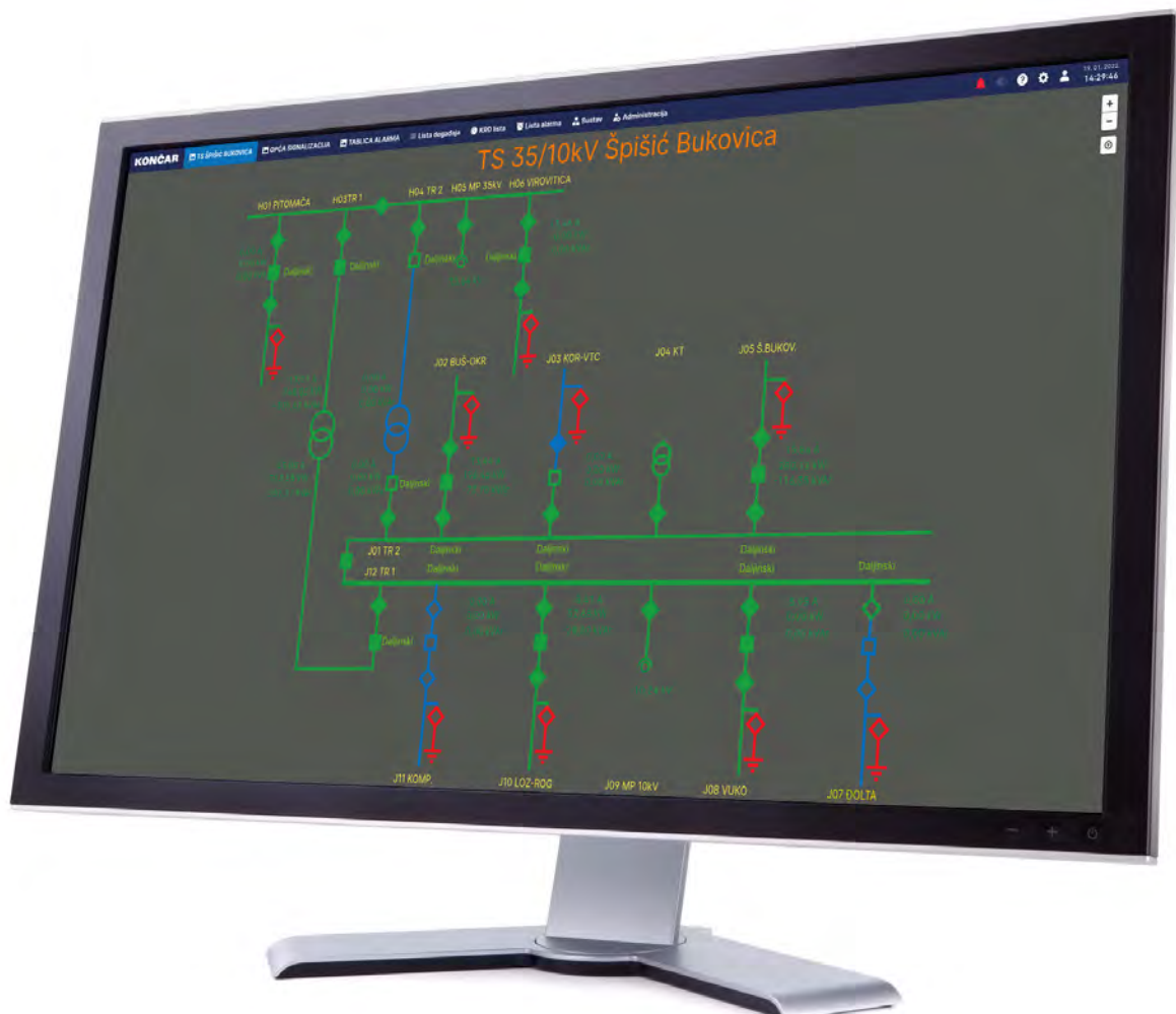
PROZA HAT EDS graphical interface
